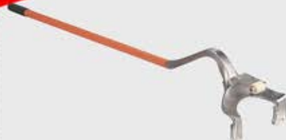
OUTIL POUR ENLEVER UN PNEU "TUBELESS"
